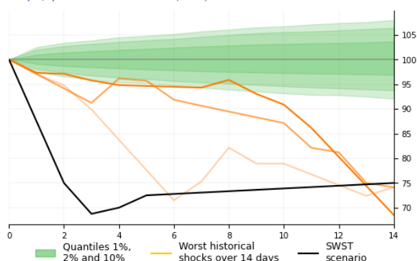
G6e: S&P 500
